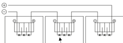
Figura 1. Serie para más voltaje
