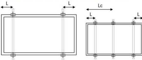
Fig. A1: Posición de las sujeciones en el marco largo
