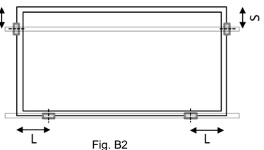
Fig. B1, B2: Posición de las sujeciones en los marcos corto y los marcos largos
