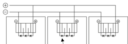
Figura 2. Paralelo para más corriente
